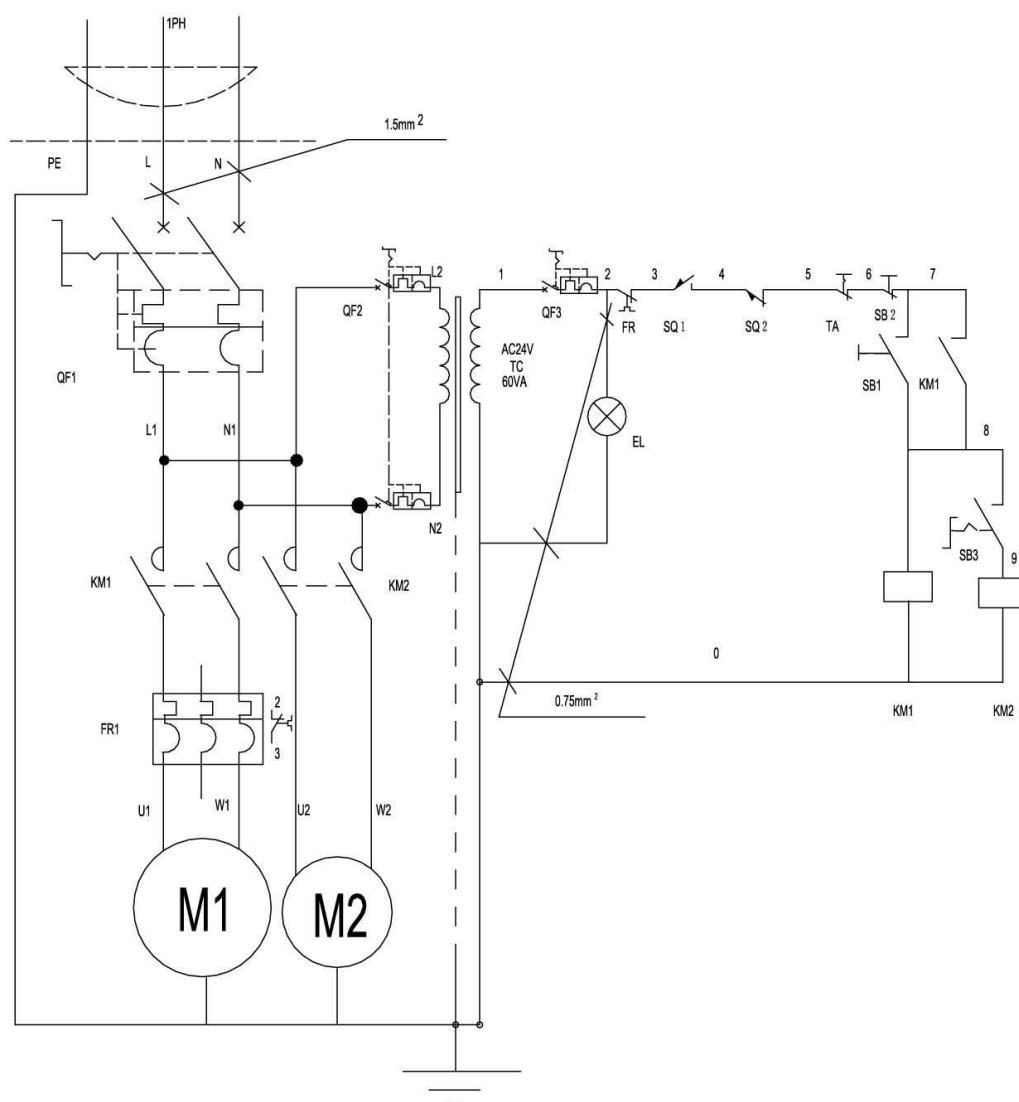
230В 50Гц 1РН А1 Спецификация электрических деталей
