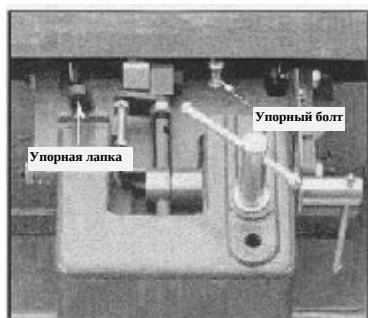
Рисунок 11. Расположение упорного болта и упорной лапки.
