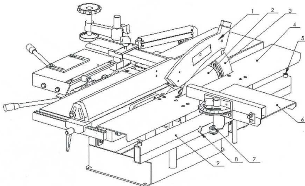
Рис. 3 Схема детали для резки
