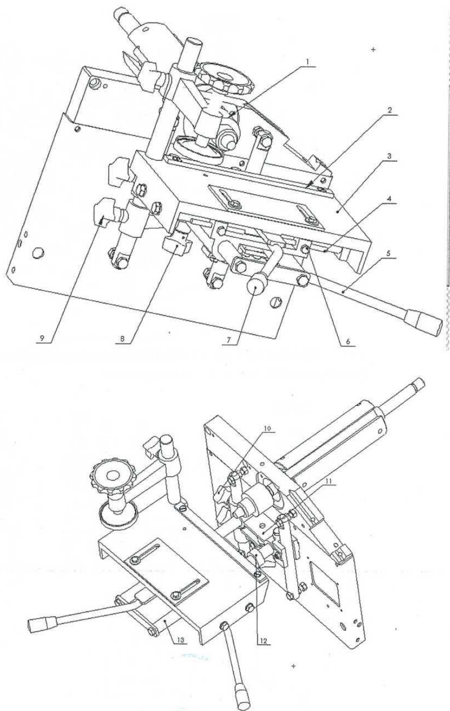
Рис. 2 Сверлильный стенд
